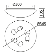
5411 Blanco-White 3L x E27 máx. 20W LED
