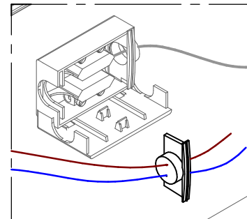
DETTAGLIO A
